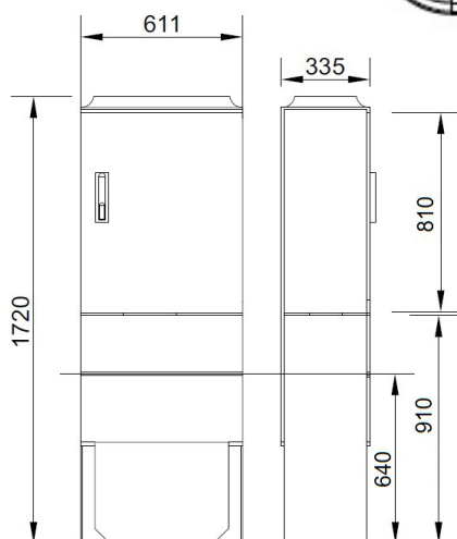
Dimensions armoire de commande (mm)
